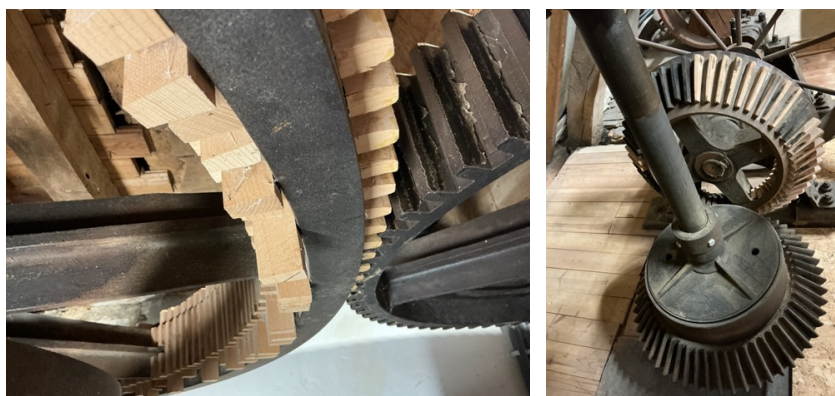
Kammen en tanden van het spoorwiel en het luiwerk.
